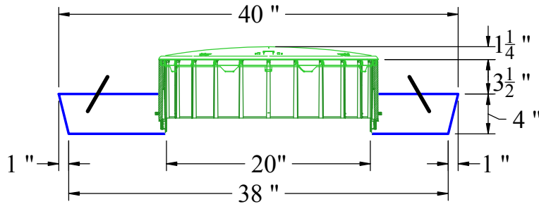
View A-A
