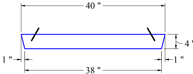
View A-A
